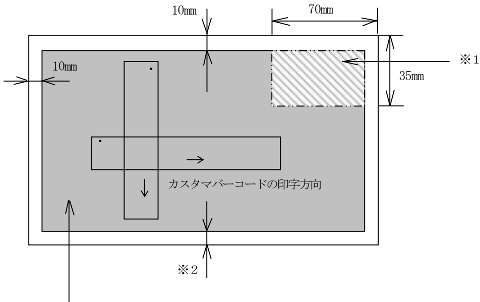
図8 カスタマバーコードの印字位置 (横に長く使用する場合の例)
