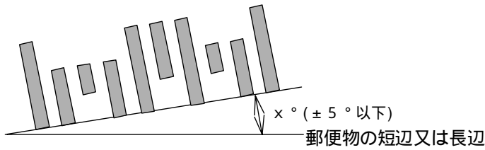
図6 カスタマバーコードの傾き
