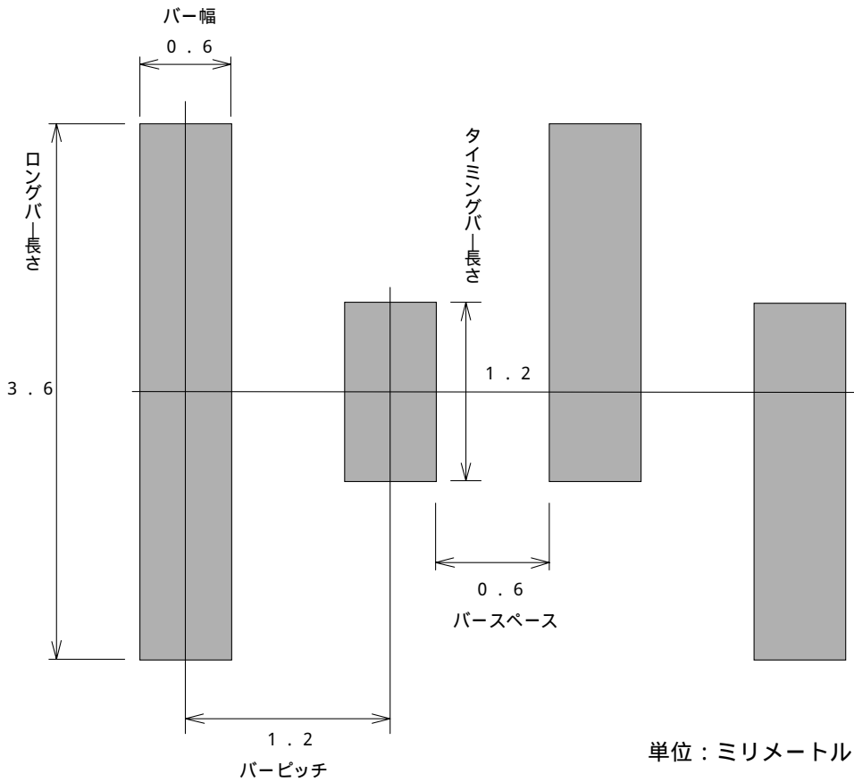
カスタマバーコードのバー基準寸法
