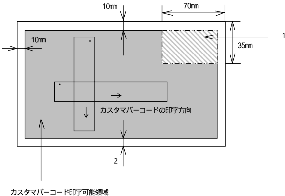
図8 カスタマバーコードの印字位置（横に長く使用する場合の例）
